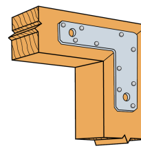
Fixation à 90° avec 66L
